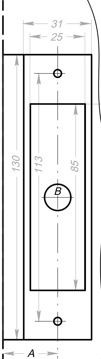
Косяк двери Door jamb
